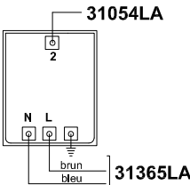
TRASFORMATEUR AC1 230VAC 25HZ COD. 88018LA
