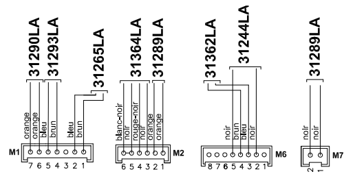
CARTE ELECTR.BMBC + DISPLAY DT - SM20019 COD. 76677LA
