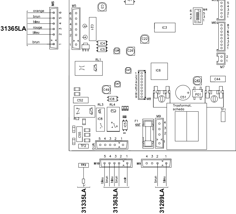
CARTE ELECTR.BMBC + DISPLAY DT - SM20019 COD. 76677LA
