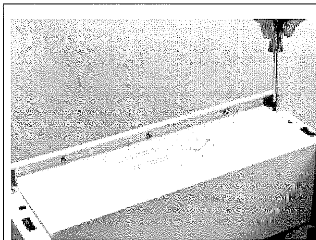
Photo A. Vis qui fixent le tableau de commande
