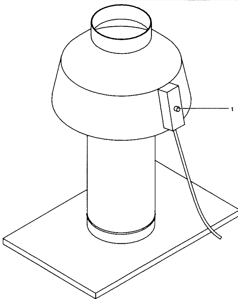
figure 4. Dispositif de coupe-tirage et anti-refouleur
