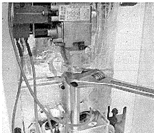
Photo L. Déconnexion groupe brûleur
